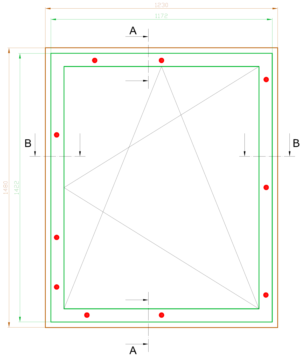
Bild 2 Ansichtszeichnung
