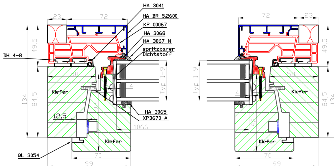
Bild 4 Horizontalschnitt, geprüft wurde mit 8 VSG SC/18/4/18/10 Verglasung (Typ 6)
