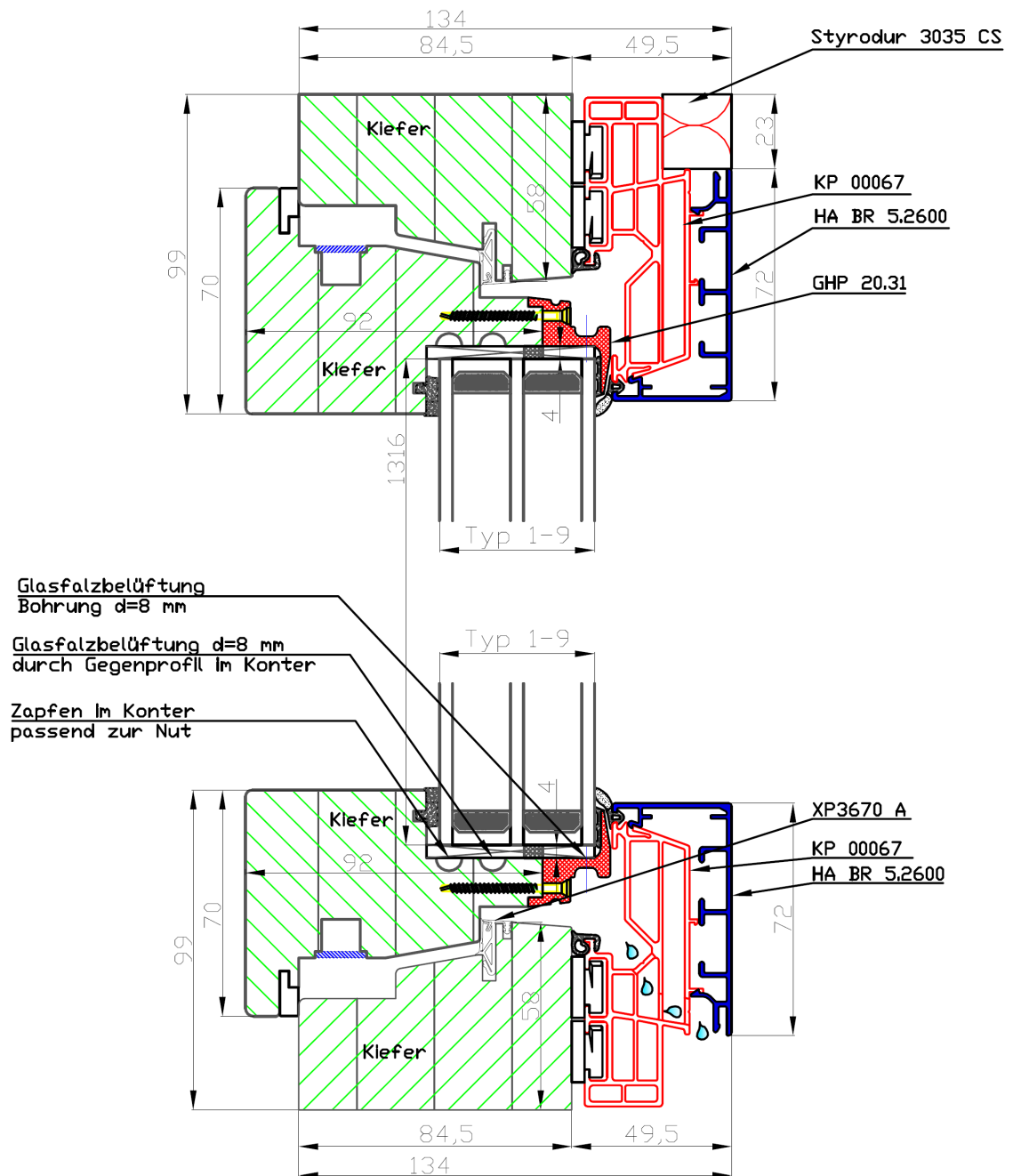
Bild 3 Vertikalschnitt, geprüft wurde mit 8 VSG SC/18/4/18/10 Verglasung (Typ 6)
